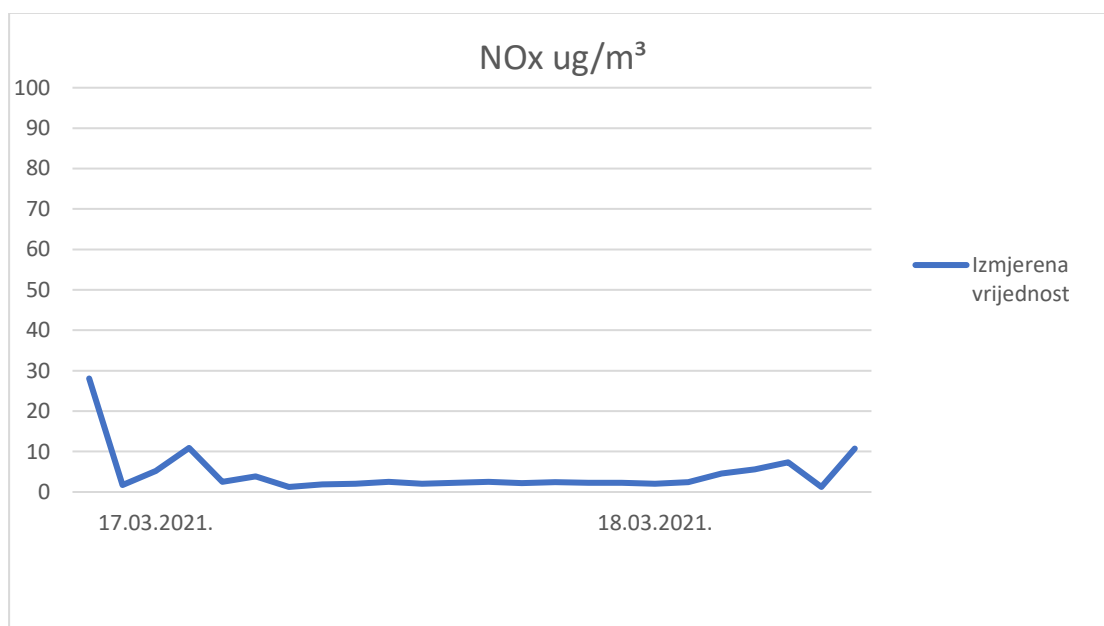
Slika 32. Grafički prikaz četveročasovnog kretanja srednjih imisijskih koncentracija NO x na lokaciji RD deponije Ubork – Buđevci
