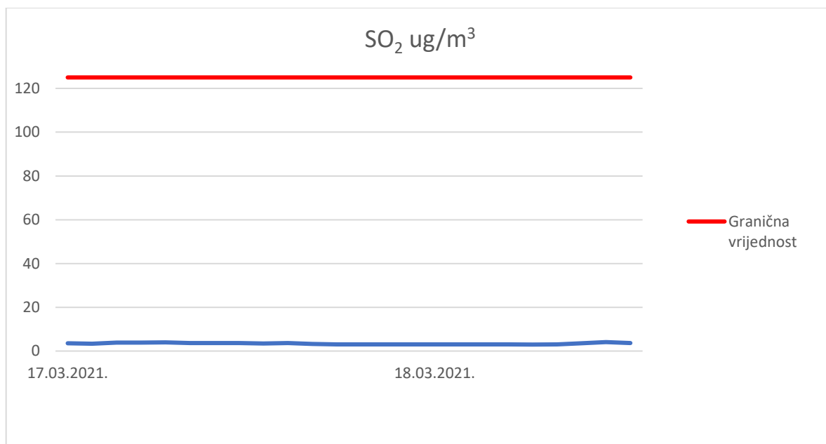
Slika 28. Grafički prikaz četveročasovnog kretanja srednjih imisijskih koncentracija SO 2 na lokaciji RD deponije Uborak – Buđevci
