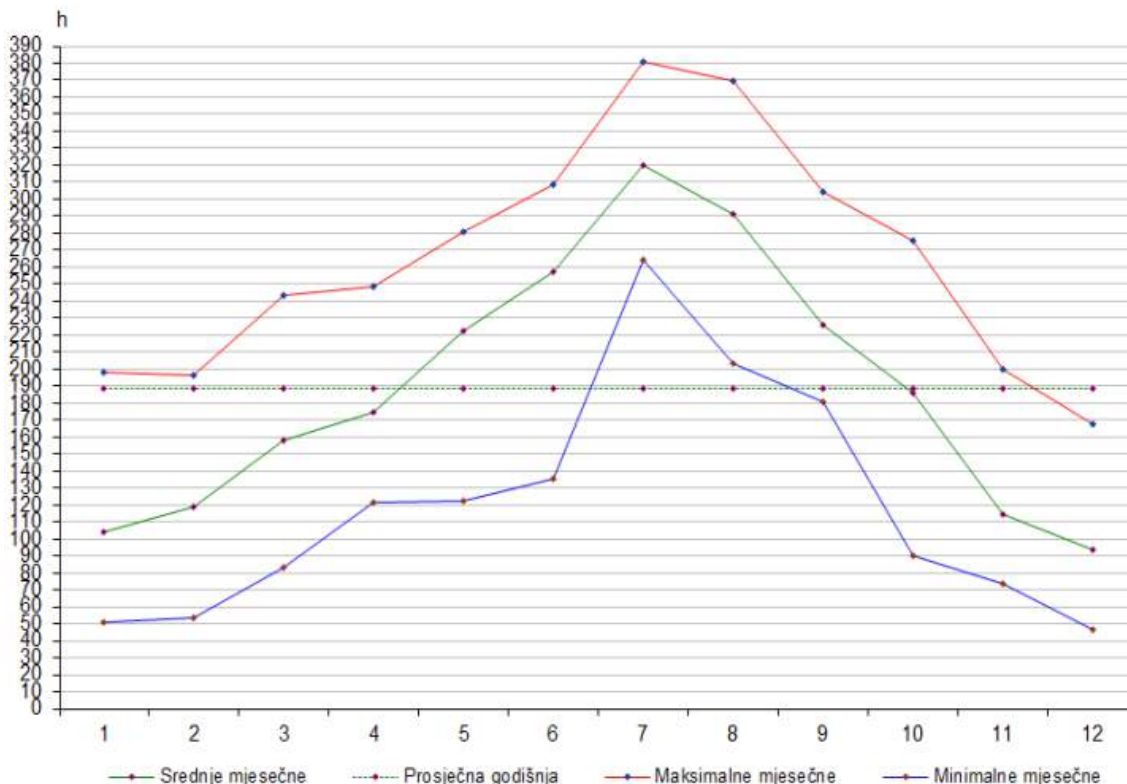
Slika 38. Godišnji tok insolacije na području Grada Mostara (Izvor: Drešković, N.: Klimatski tipovi u BiH, Doktorska disertacija, PMF Sarajevo, 2011.)
