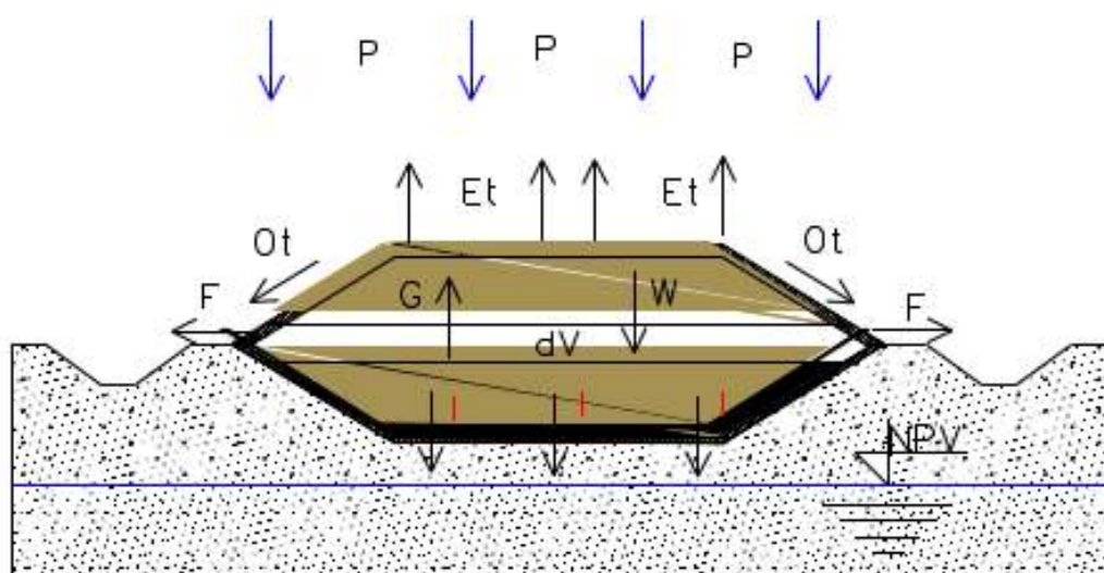
Slika 11. Elementi vodnog bilansa za deponiju
