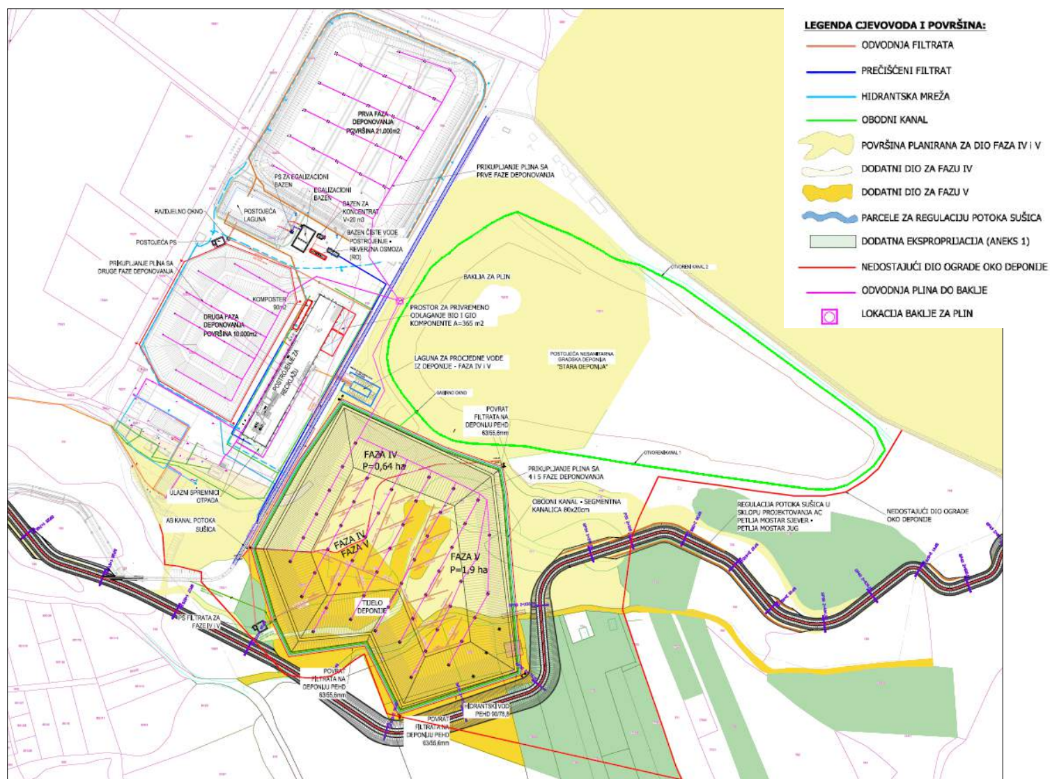
Slika 58. Kompozitna situacija projektovanog rješenja
