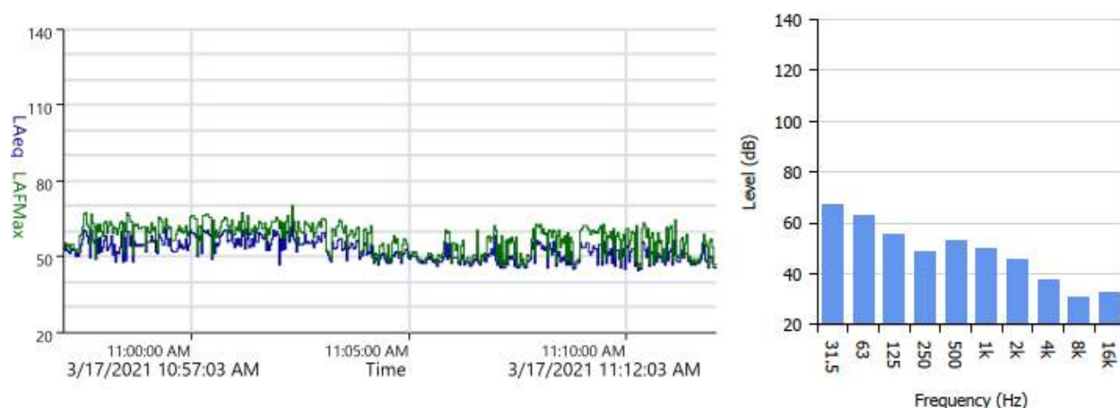
Slika 52. Grafički prikaz L_{eq} nivoa buke na lokaciji najbliže naseljene kuće u blizini Regionalne deponije Uborač – Buđevci
