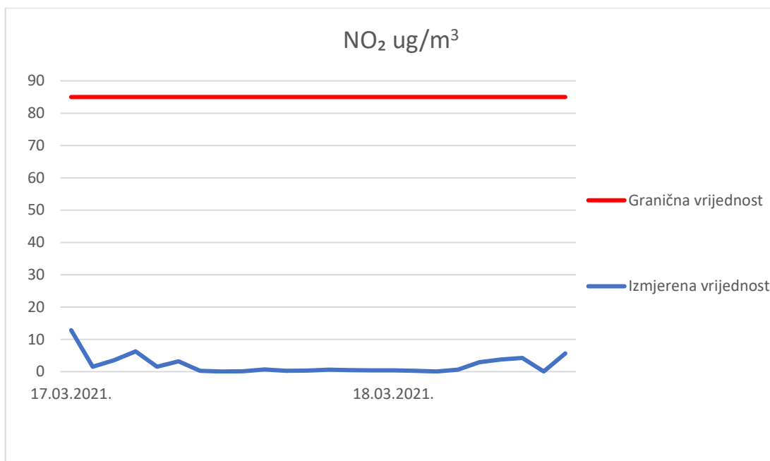
Slika 31. Grafički prikaz četveročasovnog kretanja srednjih imisijskih koncentracija NO 2 na lokaciji RD deponije Ubork – Buđevci
